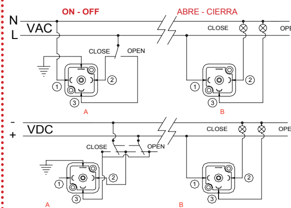
EXTERNAL ELECTRIC WIRING / ESQUEMA EXTERNO DE CONEXIONES
