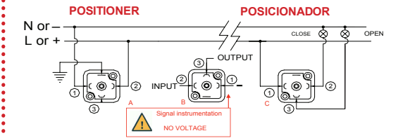
EXTERNAL ELECTRIC WIRING / ESQUEMA EXTERNO DE CONEXIONES
